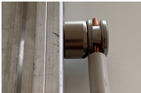
Anbindung Litzendraht an die Grundschiene Connection of stranded wire to the base trough
